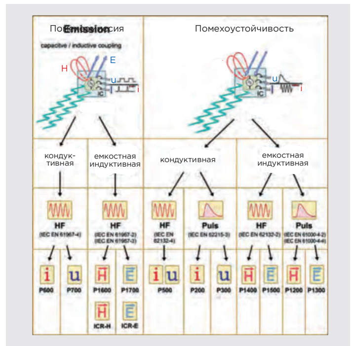
2 Группы ЭМС-стандартов для печатных плат микросхем с предложенными решениями Langer EMV-Technik по каждому из стандартов
