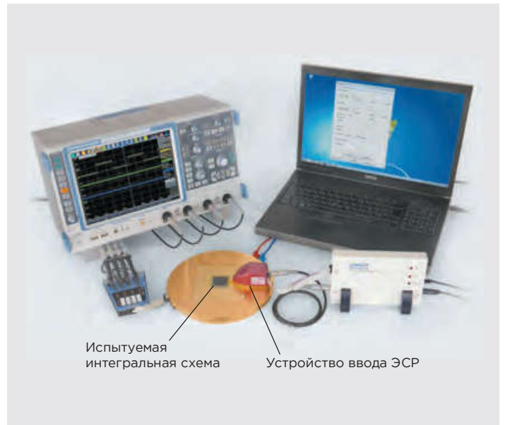
4 Установка для проведения испытаний на устойчивость к высоковольтному электростатическому разряду
