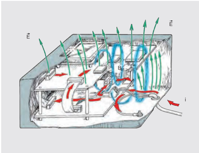
1 Распределение магнитного и электрического полей в корпусе готового устройства
