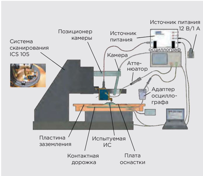
7 Система для ввода помех в микросхемы
