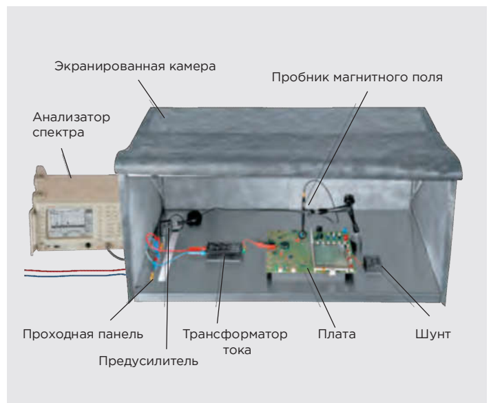
9 Установка для измерения собственного излучения печатных плат с помощью портативных пробников
