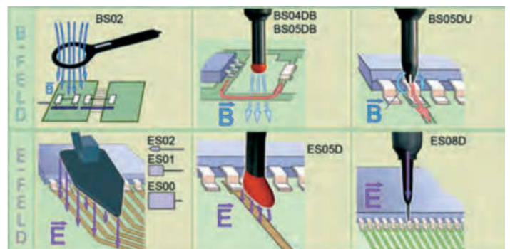
6 Портативные инжекционные пробники Langer EMV-Technik
