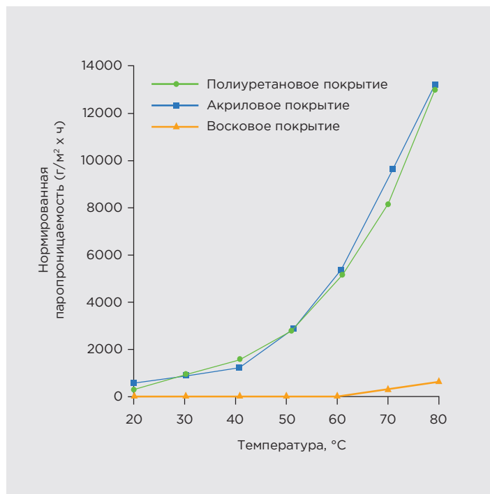
Паропроницаемость влагозащитных покрытий
