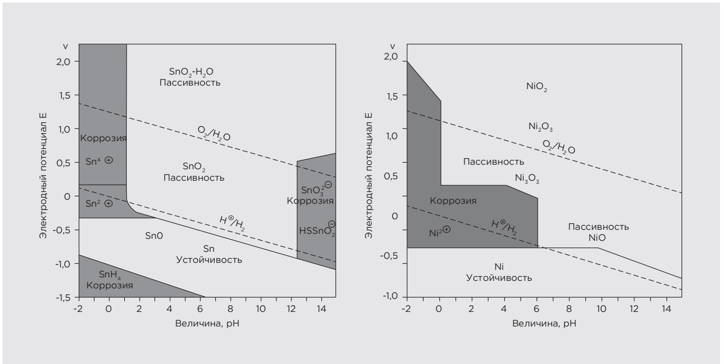
7 Диаграмма Пурбе для олова и никеля
