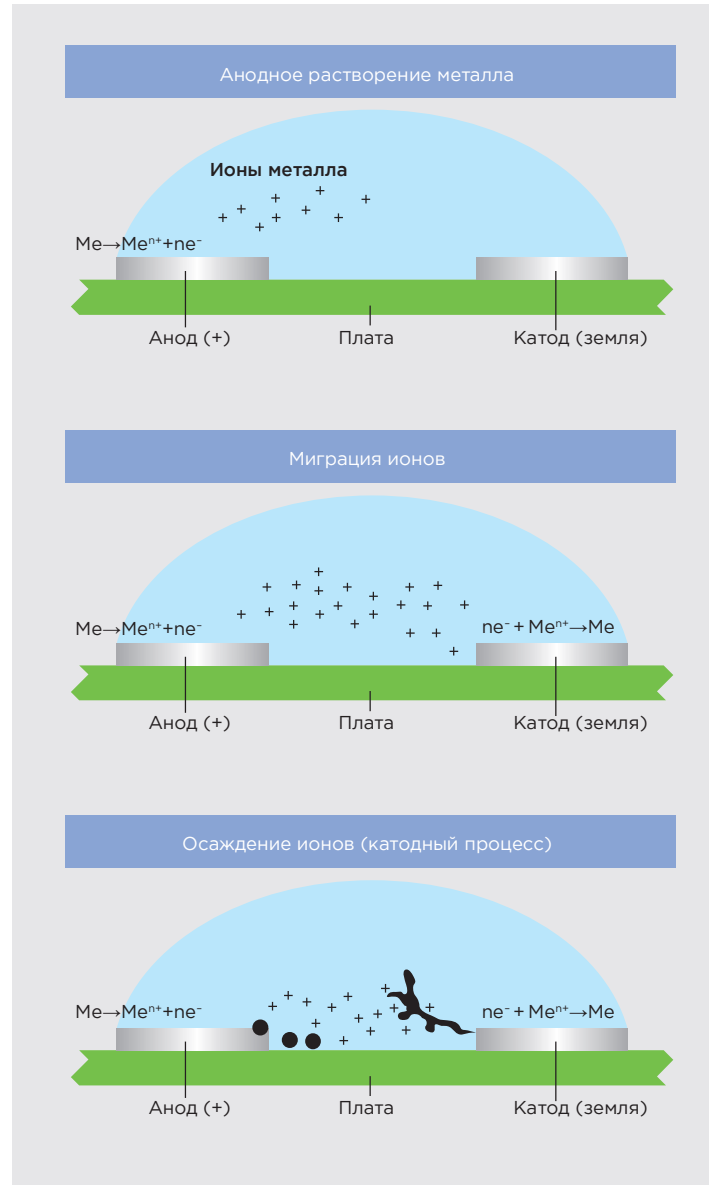
2 Схематическое представление механизма возникновения электрохимической миграции
