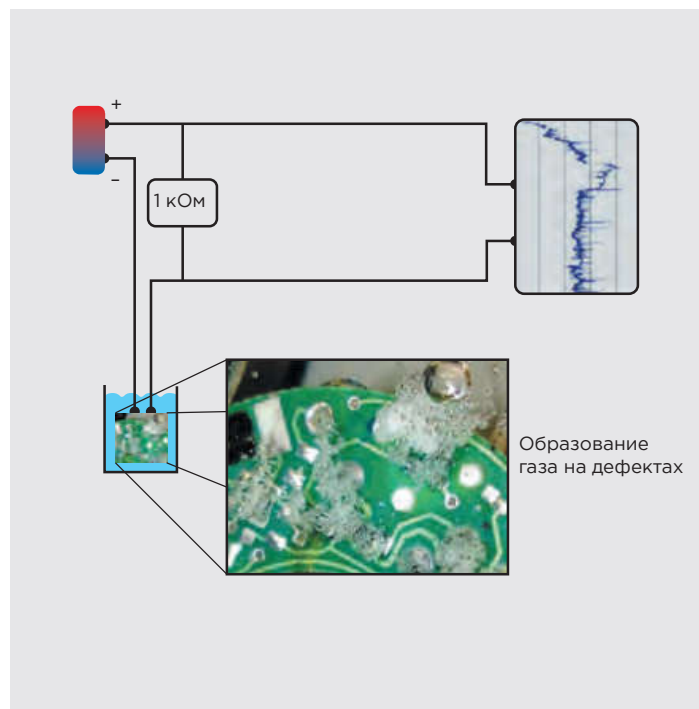
Схема проведения CORE-теста
