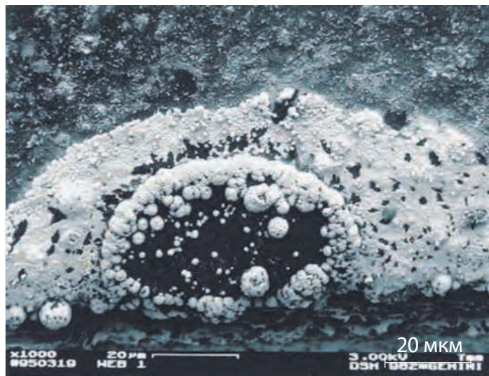
Коррозия, вызванная коррозионными газами
