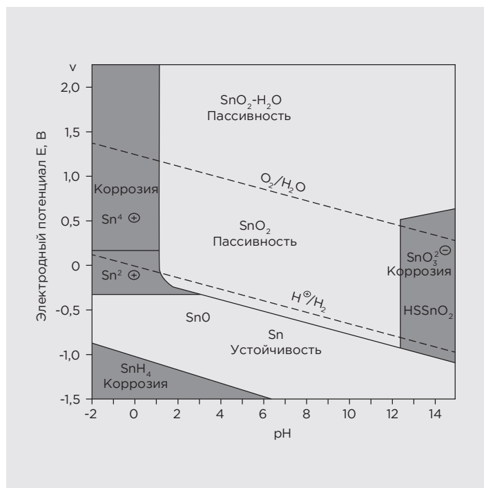
Диаграмма Пурбе для олова
