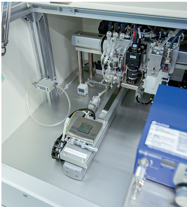
Система STM-II автоматизированной установки шариковых выводов от компании Shinarex
